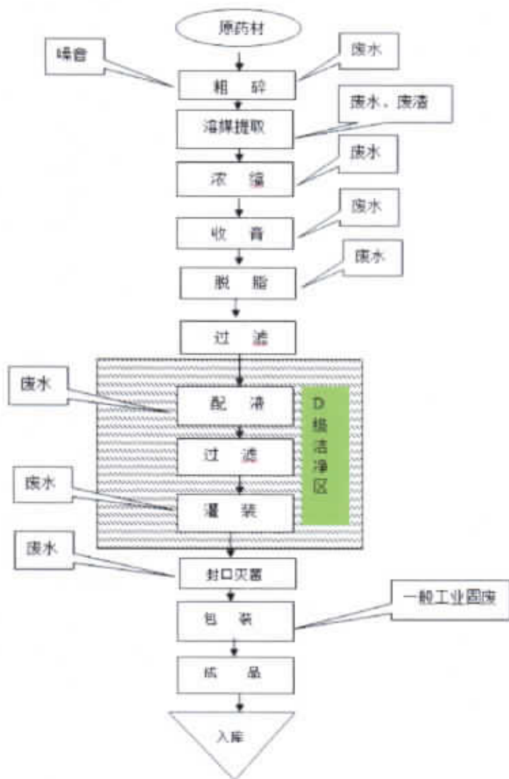
图 3-1 康复新液生产工艺流程图
