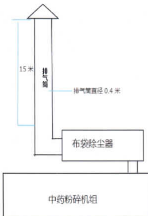
图 3-6 前处理提取车间粉碎间废气处理工艺流程图
