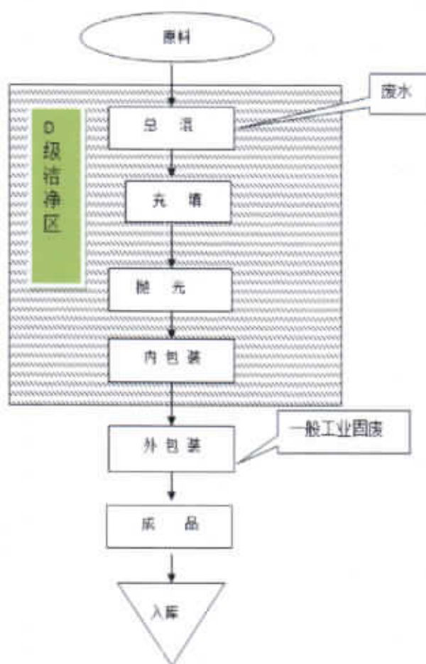
图 3-2 胶囊剂生产工艺流程图
