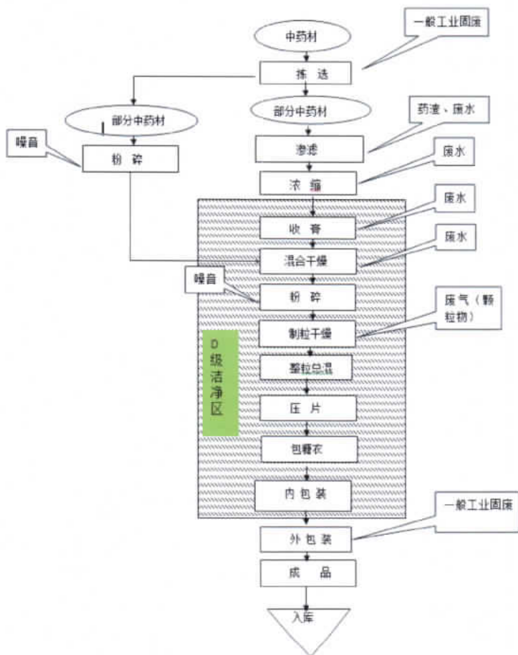
图 3-4 片剂生产工艺流程图
