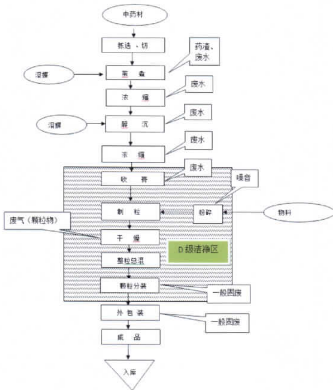
图 3-3 颗粒剂生产工艺流程图
