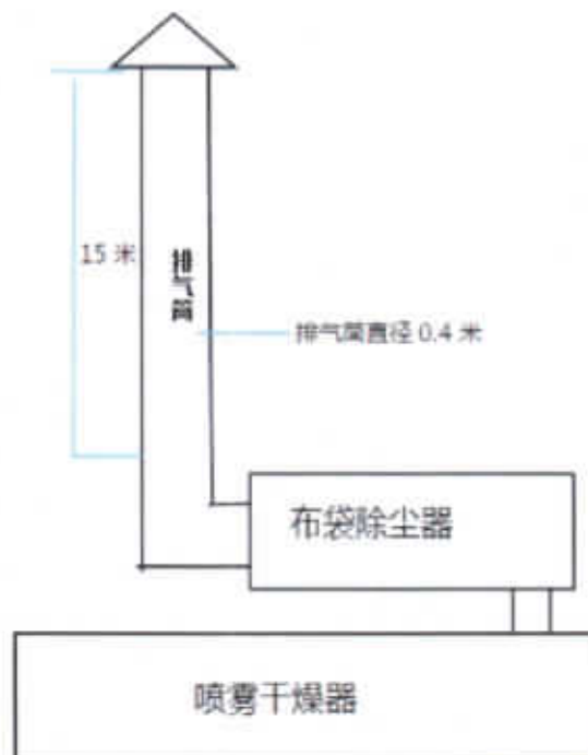
图 3-8 固体制剂喷雾干燥器废气处理工艺流程图
