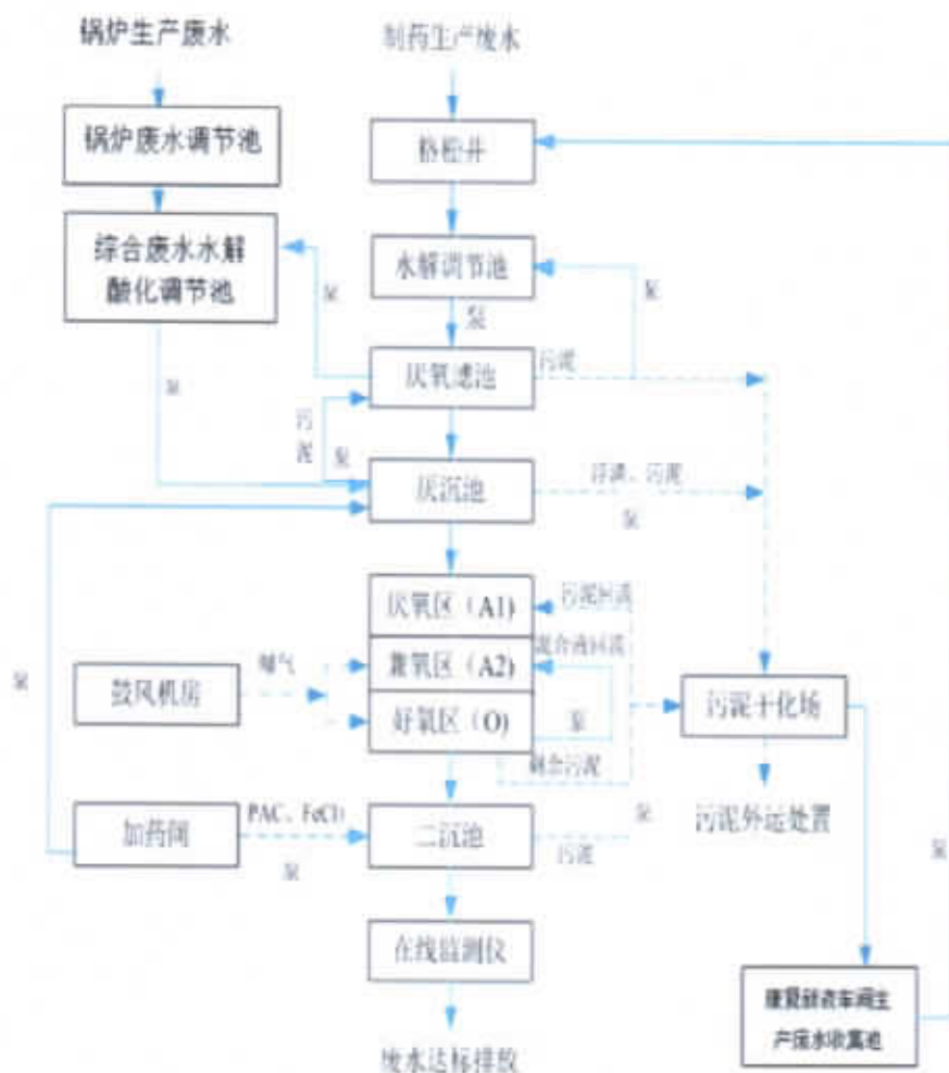
图 3-5 污水处理系统工艺流程图
